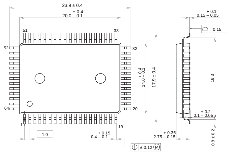
64PIN QFP(PLASTIC)
